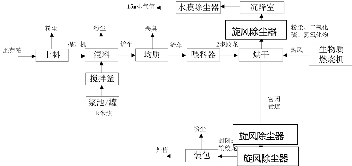
生产工艺流程及产污环节图
