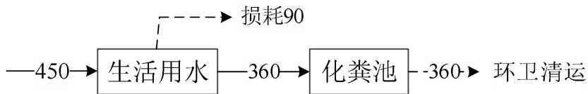
项目新鲜水用水平衡图 ( \text{m}^3/\text{a} )
