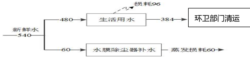
项目水平衡图 单位 \text{m}^3/\text{a}
